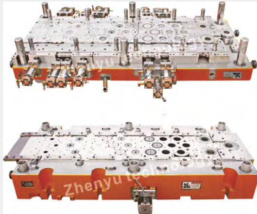
定转子铁芯级进模具 progressive lamination die
