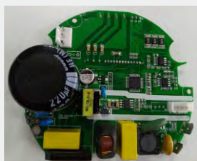
Ec风机无刷电机控制器 EC fan brushless motor controller
