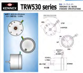
TRW530 马达 TRW530 motor
