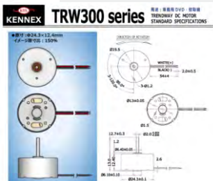
TRW300马达 TRW300 motor
